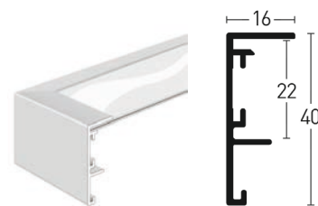
Max. Einlegehöhe 20 mm | Max. insertion height 20 mm
