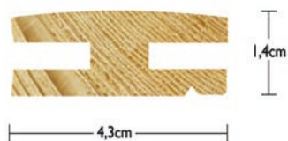
Mittelstrebe | Centre strut
